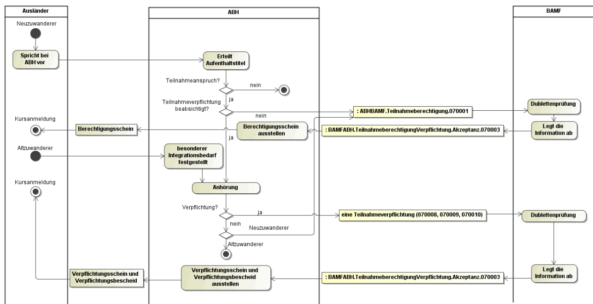
Abbildung 6.18. „Einfacher Ablauf“ bei Teilnahmeberechtigung/-verpflichtung
