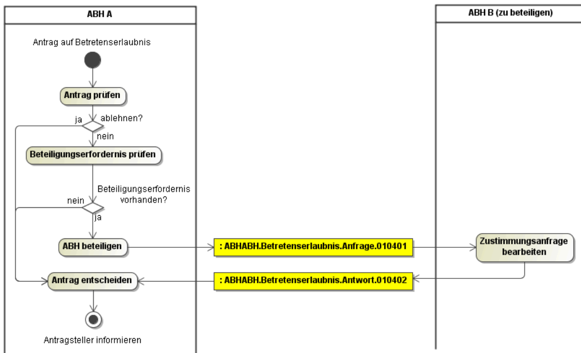
Abbildung 3.15. Das Aktivitätsdiagramm Betretenserlaubnis
